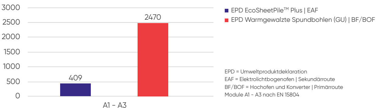
Treibhausgaspotenzial [kg CO 2 e / t Spundbohle]
