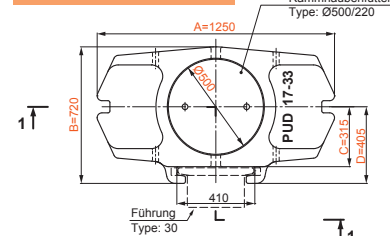
Draufsicht [mm]
