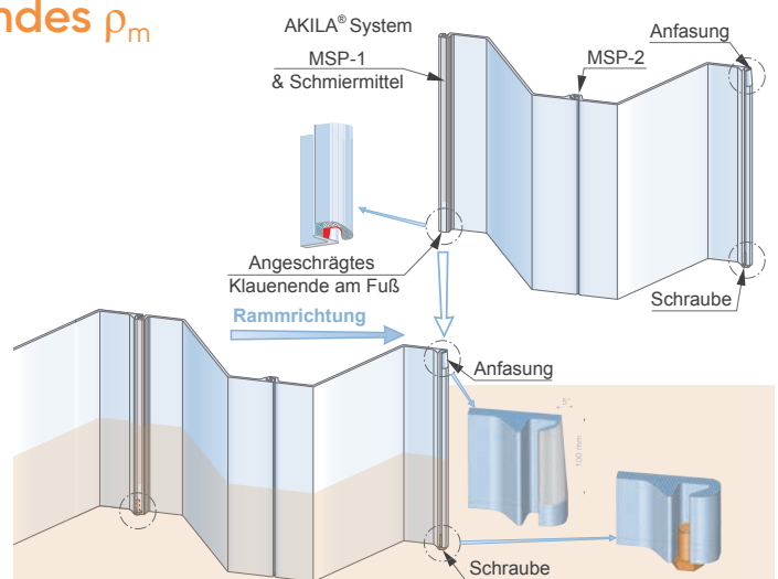
Rammhinweise (Rammrichtung, Anfasung usw.).
