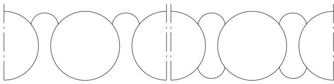
Kreiszellen mit 35^\circ Abzweigbohlen und einer Zwickelwand oder zwei Zwickelwänden.
