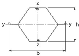
Z-Pfahlprofil
