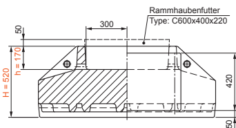
Schnitt 1-1 (UZD 14-28) [mm]
