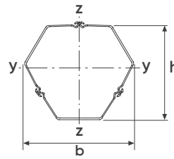
U-Dreifachpfahlprofil
