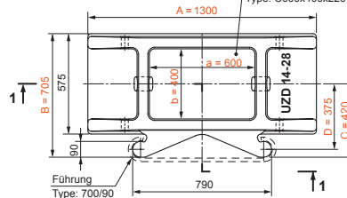
Draufsicht [mm]
