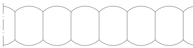
Flachzellen mit 120^\circ Abzweigbohlen.
