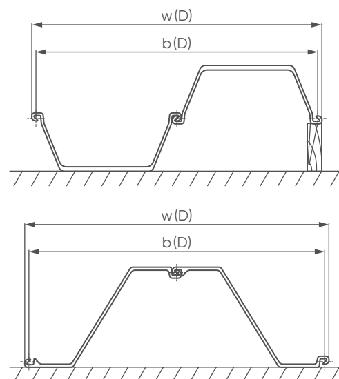
Beispiel für Doppelbohlen
