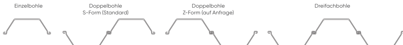
Doppelbohle S-Form (Standard)
